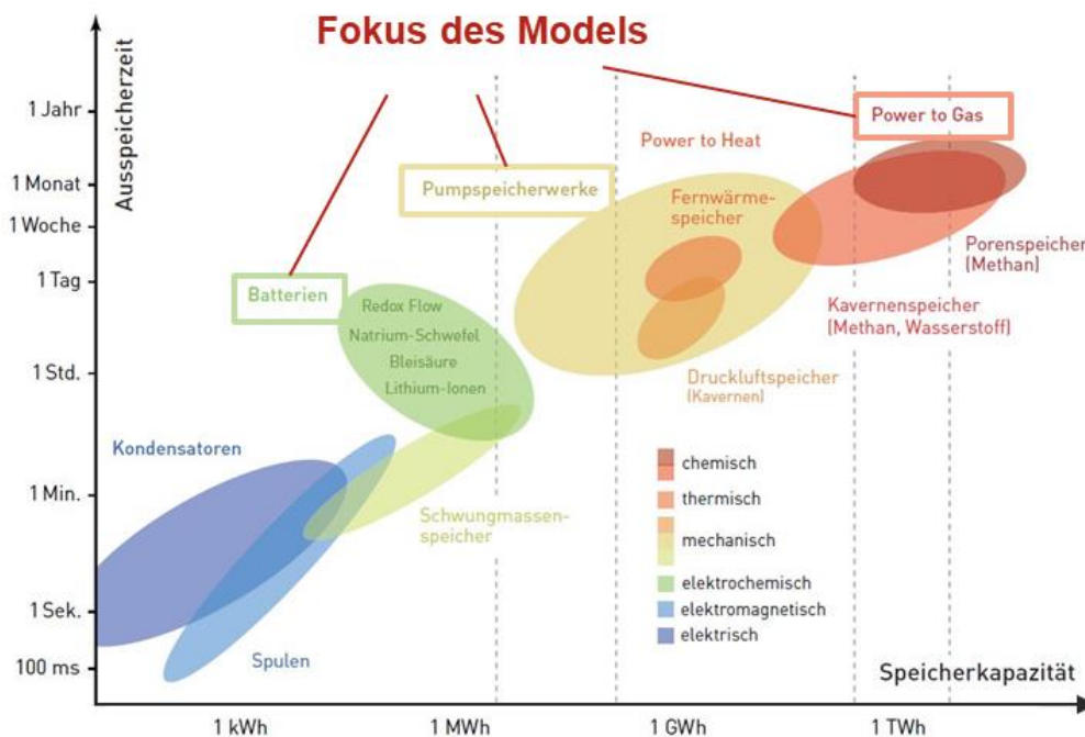
Abbildung 4 Übersicht über unterschiedliche Speichertypen (Frontier Economics, 2017), (Stern et al. 2014 zit. nach (Frontier Economics, 2017)), Navigant Analyse
