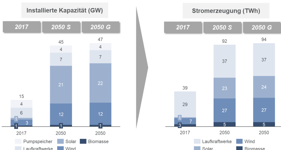
Abbildung 7: Installierte Kapazität (links) und Stromerzeugung (rechts) für die Jahre 2017, 2030 und 2050 für das Strom- und Gasszenario. Summen gerundet.
